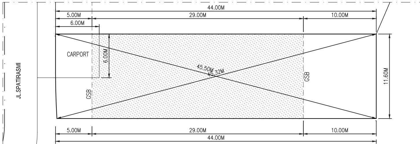
DENAH UNIT HUNIAN JL.SPATIRASMI NO. 71 SKALA 1 : 300
