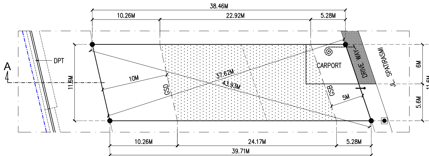
DENAH UNIT HUNIAN JL. SPATIRASMI NO.92 SKALA 1 : 350
