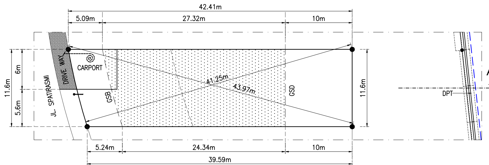
DENAH UNIT HUNIAN JL. SPATIRASMI NO.75 SKALA 1 : 350
