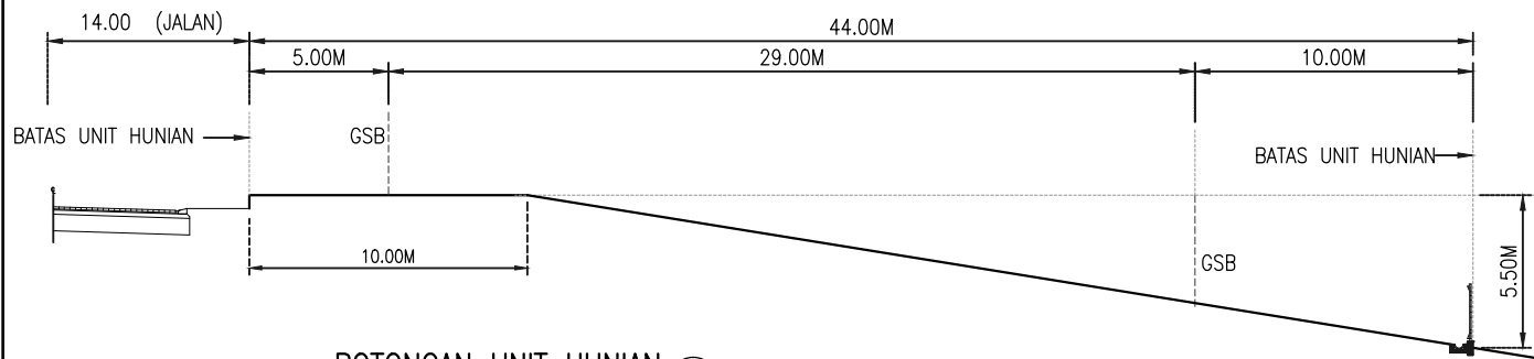
POTONGAN UNIT HUNIAN SKALA 1 : 300
