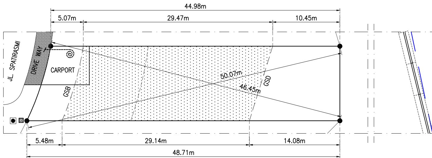
DENAH UNIT HUNIAN JL. SPATIRASMI NO.107 SKALA 1 : 400
