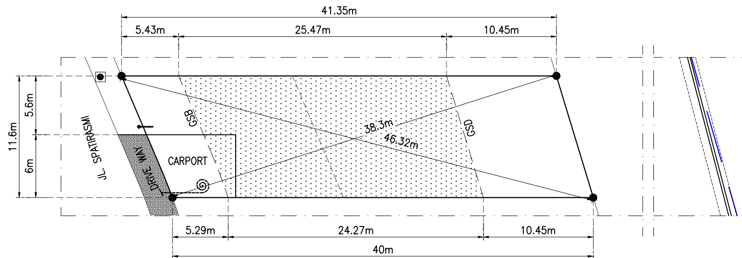
DENAH UNIT HUNIAN JL. SPATIRASMI NO.101 SKALA 1 : 400
